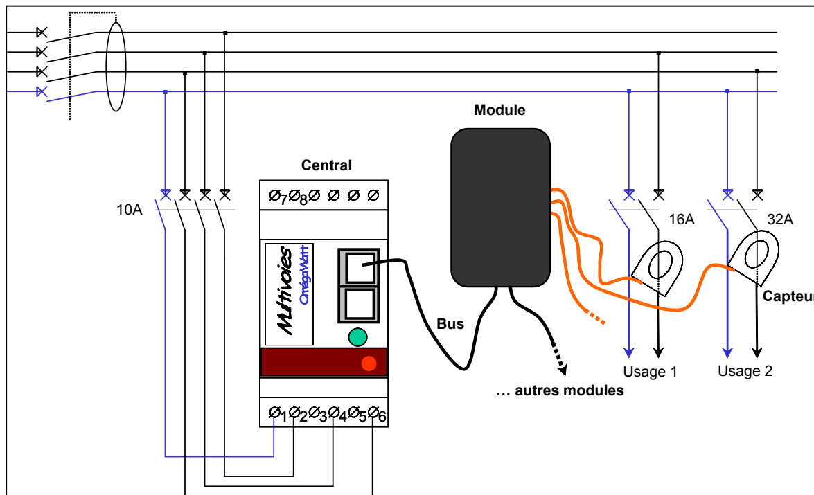
Schéma de branchement dans un tableau triphasé
